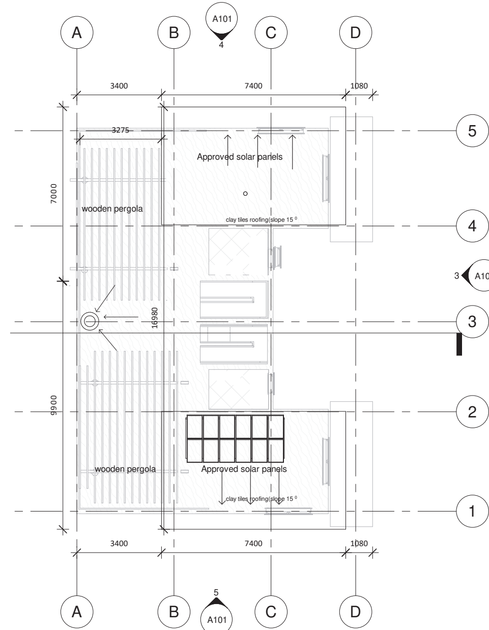
SEMI-DETACHED MAISONETTE ROOF PLAN SCALE 1:100
