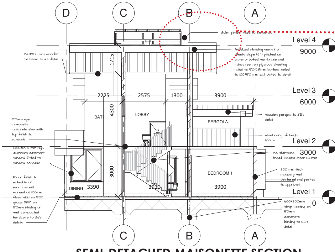
SEMI-DETACHED MAISONETTE SECTION SCALE 1:100
